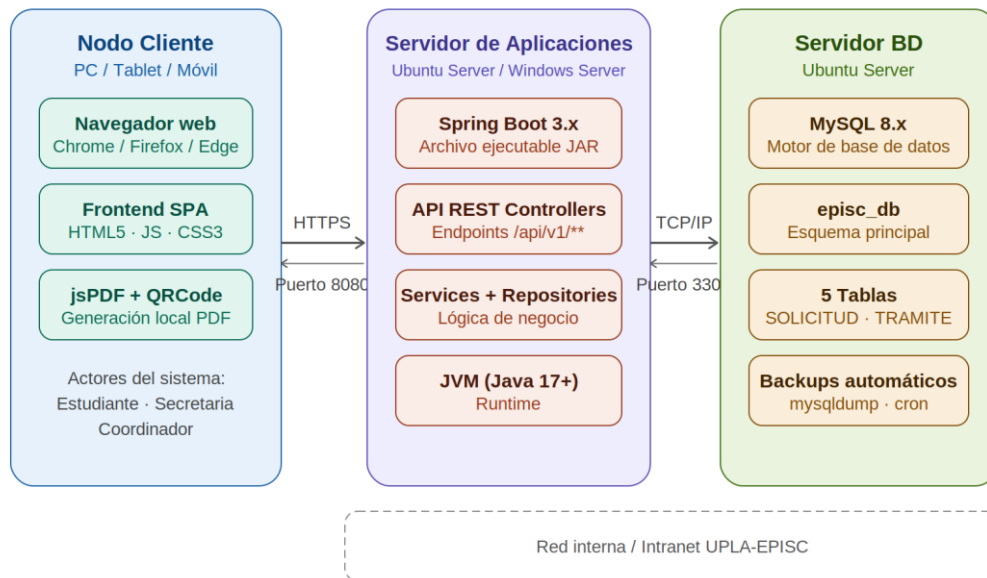
Figura 1.2: Diagrama de Despliegue del Sistema
