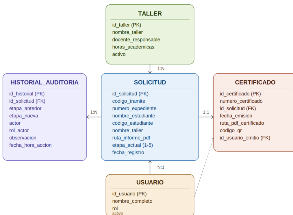
Figura 1.3: Diagrama Entidad-Relación de la Base de Datos
