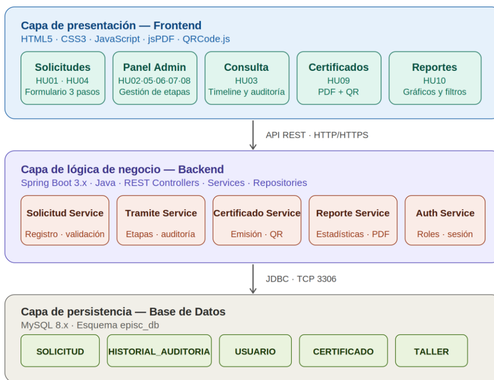
Figura 1.1: Diagrama de Componentes del Sistema
